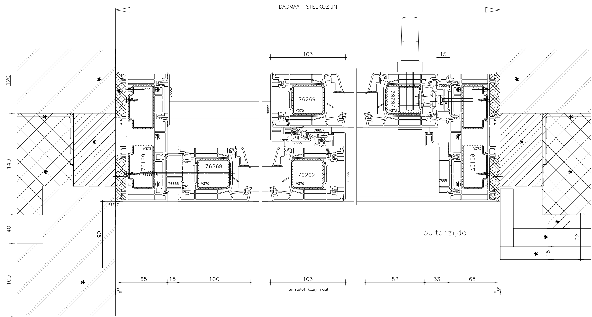
DOORSNEDE A-A
