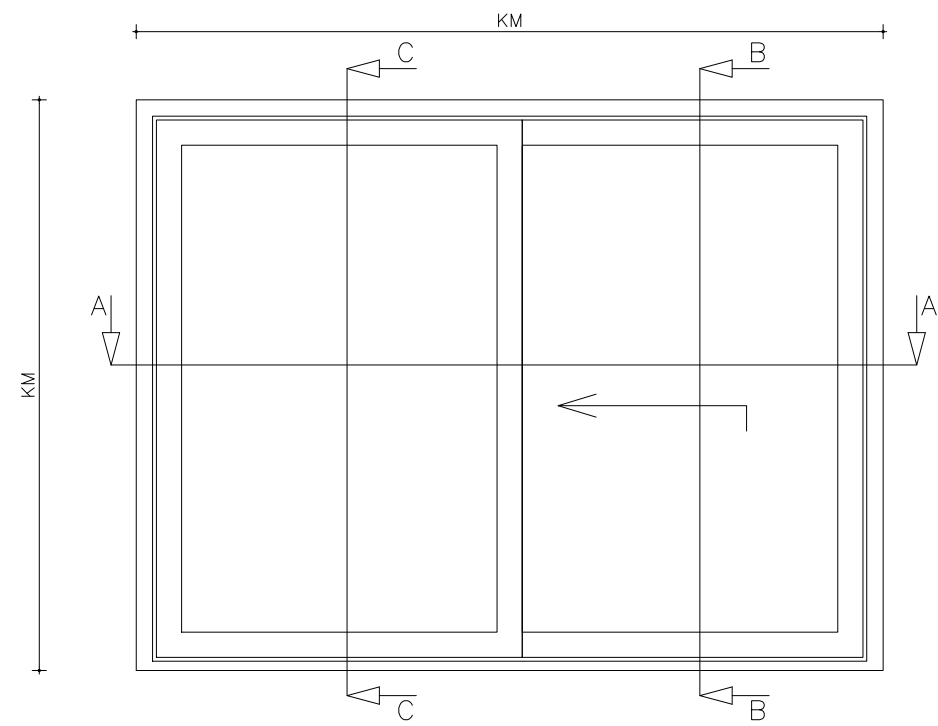
BUITENAANZICHT
