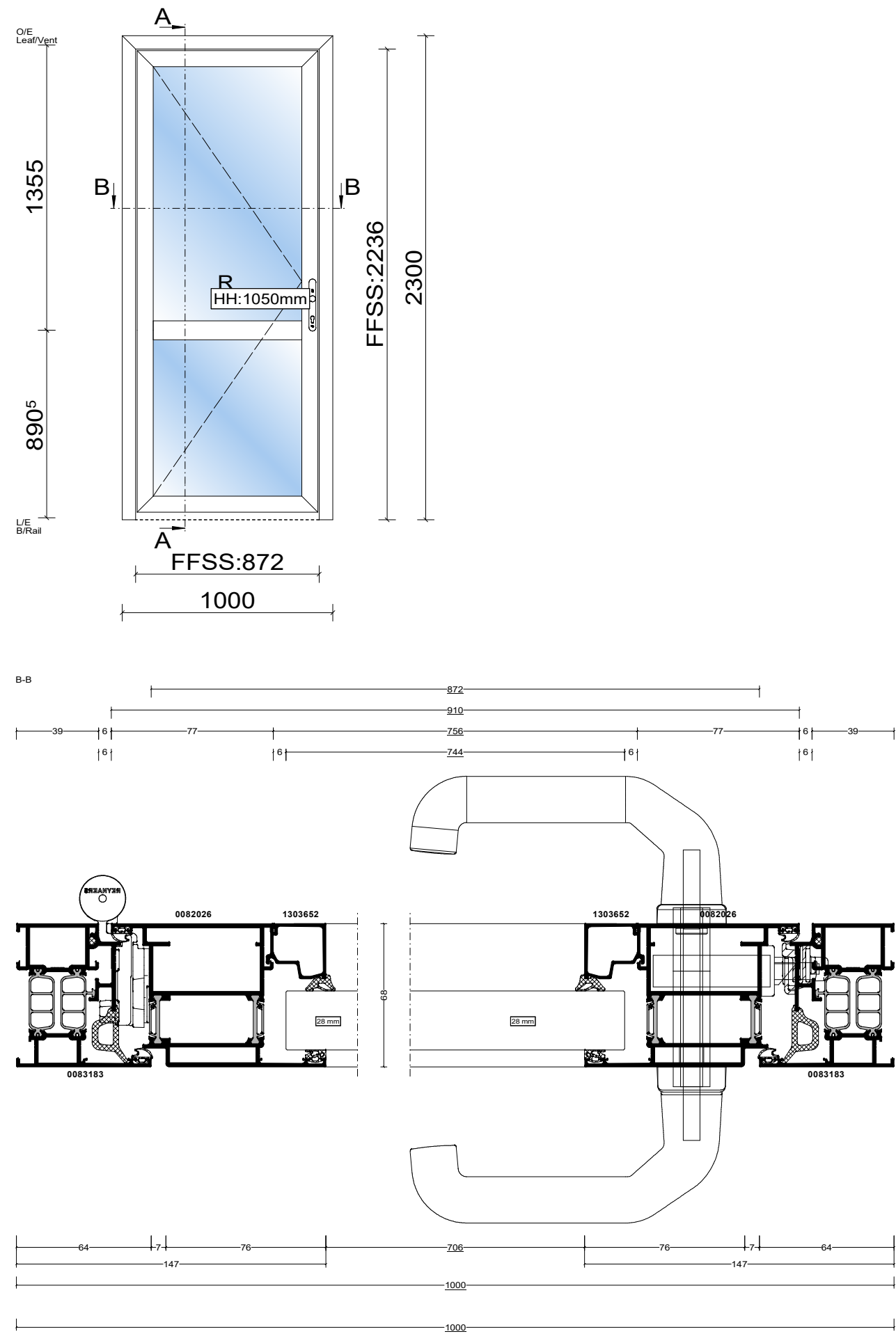
Reynaers CS77 TK02 voordeur (binnendraaiend)
